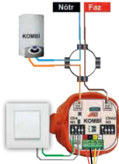
KOMBİ BAĞLANTISI
