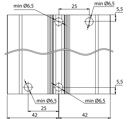
Koruma kapağı delik şablonu!
