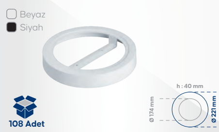
LP12 12W Sıva Üstü Led Panel Kasası
